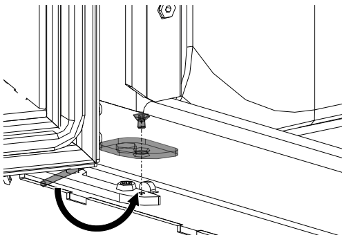
Abb. 26: Tür einhängen und Feder spannen
