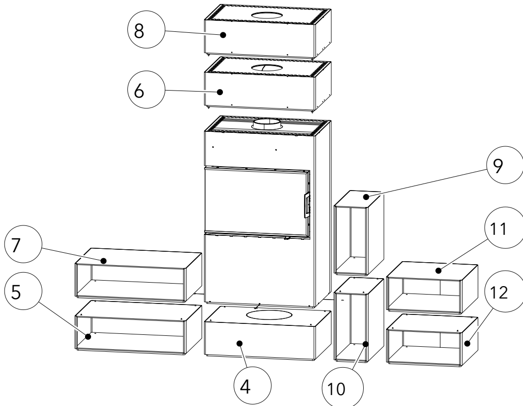
Abb. 24: Beistellboxen
