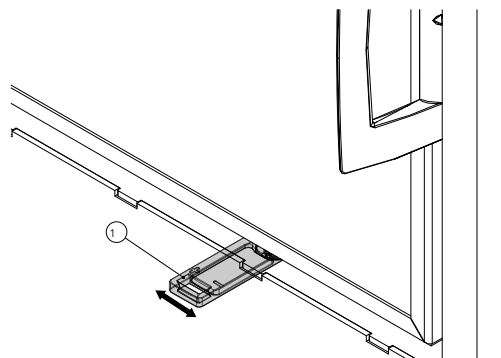
Abb. 31: Primär- Sekundärluftschieber
