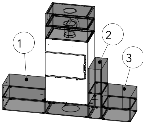
Abb. 23: Beistellboxen
