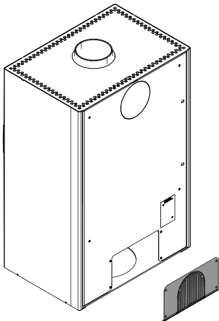
Abb. 10: Revision demontieren
