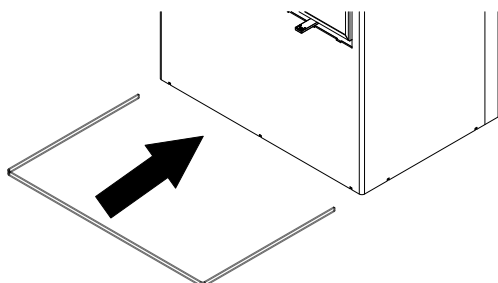
Abb. 9: Schattenfuge einlegen
