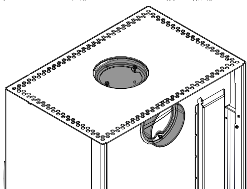
Abb. 15: Abdeckung und Stutzen tausche
