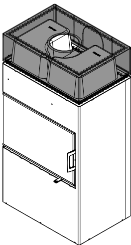
Abb. 21: Aufsatzbox auf HMS-Steine
