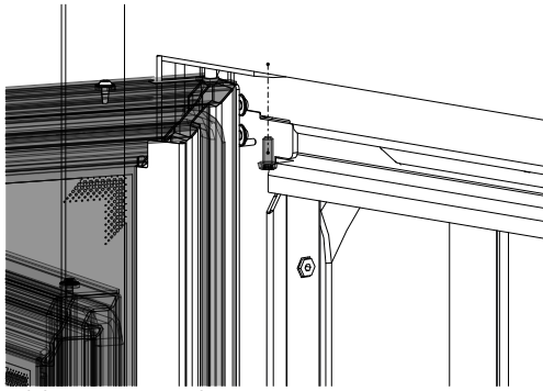
Abb. 25: Tür einhängen
