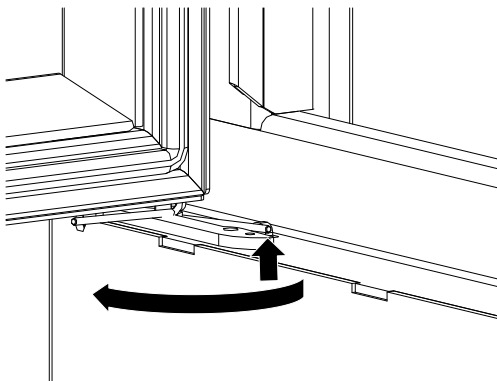
Abb. 42: Feder lösen
