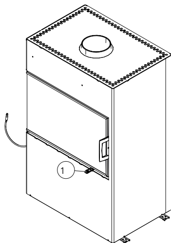
Abb. 4: Luftregler
