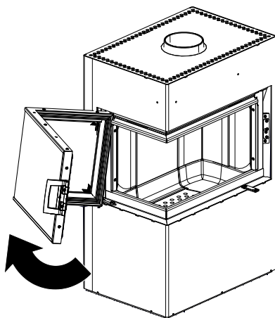
Abb. 43: Tür aushängen
