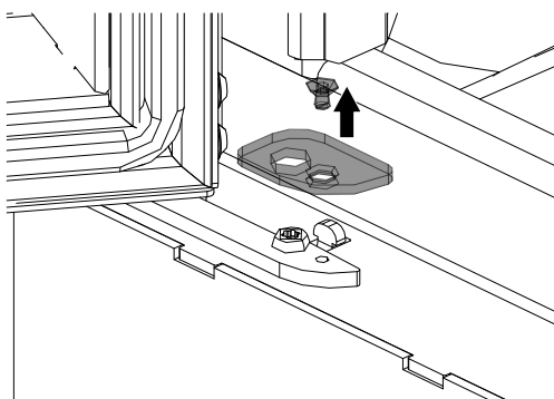
Abb. 41: Federabdeckung lösen
