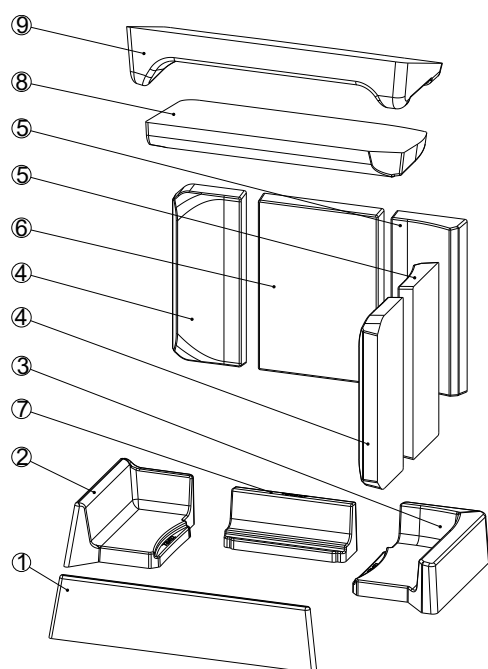
Abb. 19: Keramott
