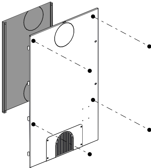
Abb. 12: Strahlenschutz demontieren
