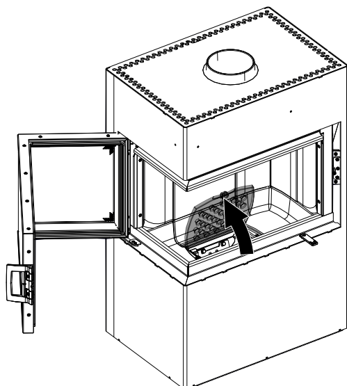
Abb. 34: Rost hochklappen
