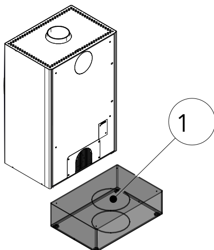
Abb. 17: Sockel mit Ausschnitt
