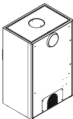
Abb. 16: Rückwand montieren
