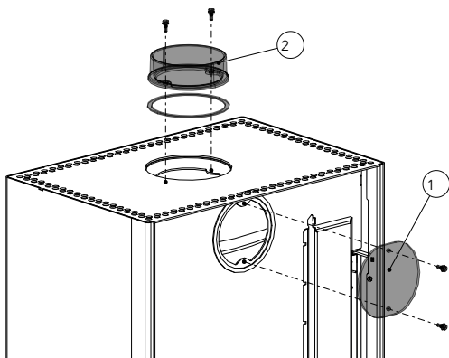
Abb. 14: Abdeckung und Stützen demontieren
