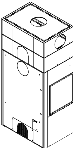
Abb. 22: Aufsatzboxen auf HMS-Steine
