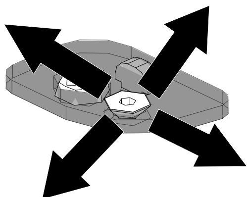
Abb. 30: Tür einstellen
