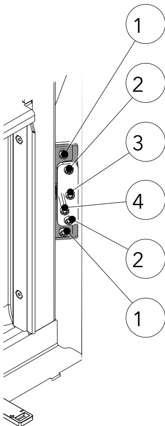
Abb. 28: Türverschluss einstellen
