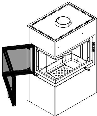
Abb. 29: Tür öffnen
